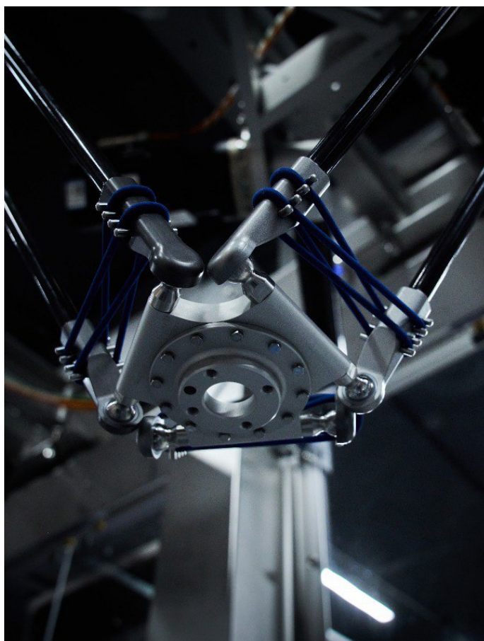
Дельта-робот.
