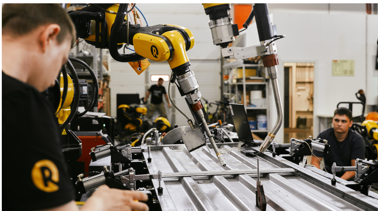
Роботизированная сварочная ячейка A12-PVHN-600.
